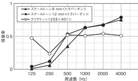
図3 岩綿吸音板 吸音性能
