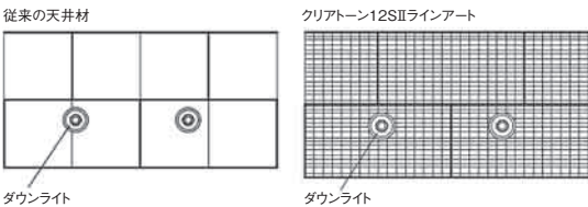
図2 クリアトーン12SⅡライアンアート 照明配置図
