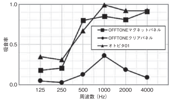
図7 後付け吸音パネル 吸音性能
