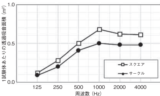
図6 KIN TONE(キントーン)吸音性能
