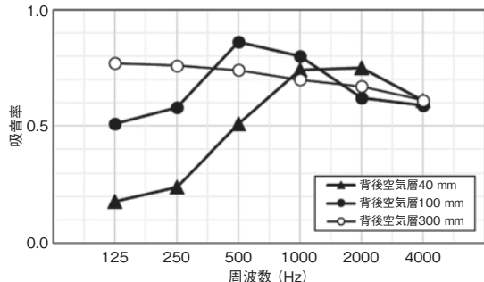
図5 スオーノ 吸音性能
